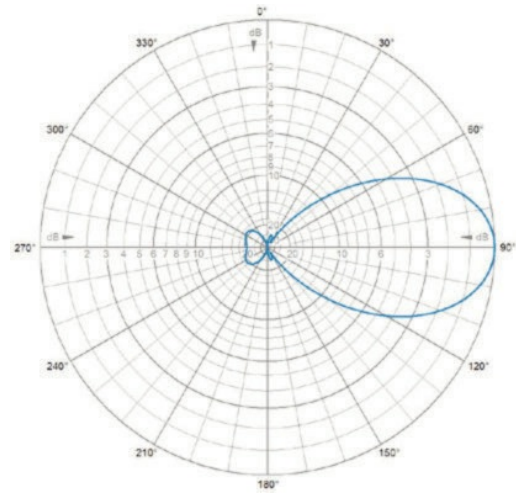
E-Plane | 165 MHz
