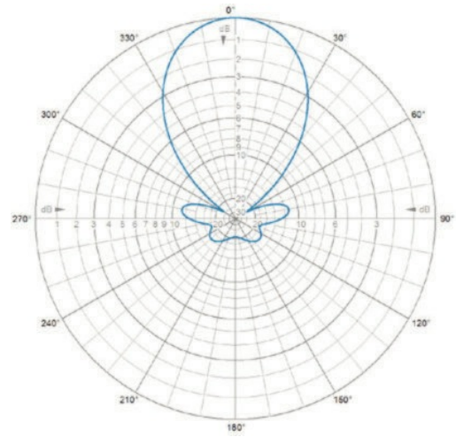
H-Plane | 165 MHz
